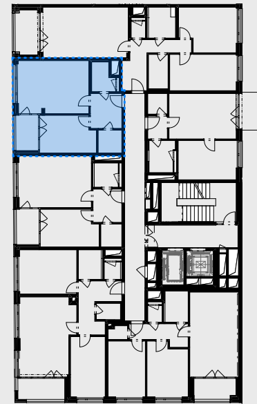
Půdorys podlaží
